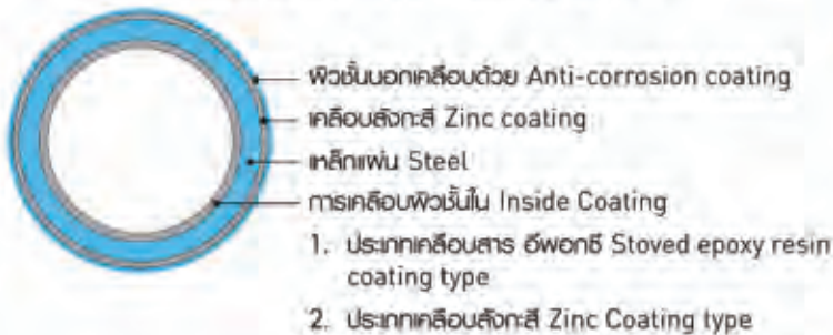
ภาพรูปตัดด้านข้างของท่อร้อยสายไฟฟ้า
